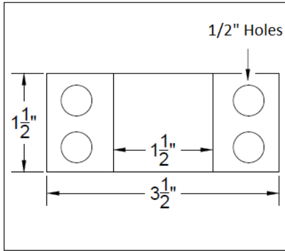
2 SECTION DETAIL: A-A
